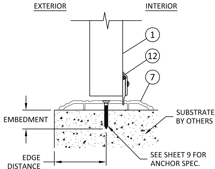
H 6 VERTICAL SECTION INSWING DOOR SILL
